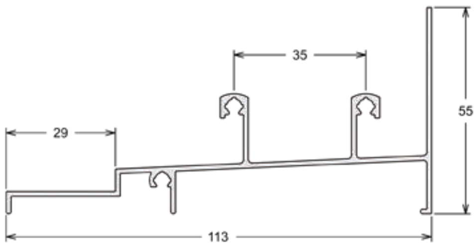
IT-003 | PESO: 5,600 KG/BR Marco Inferior Horizontal
