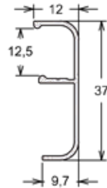
MP-348 | PESO: 1,300 KG/BR Arremate / Vista Interna
