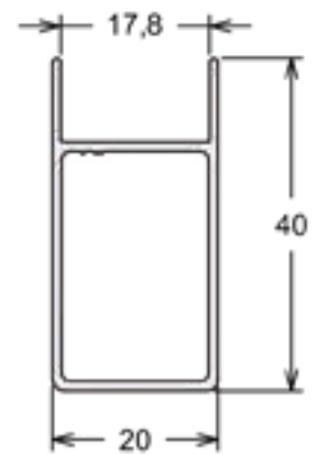
MP-305 | PESO: 2,300 KG/BR Folha Lateral Vertical - Veneziana
