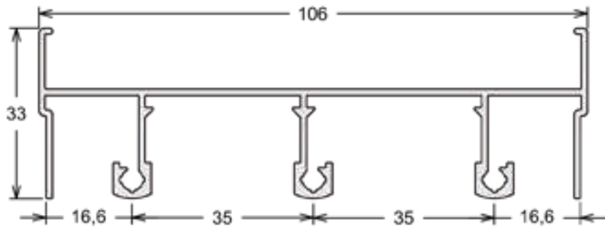
SU-010 | PESO: 5,800 KG/BR
