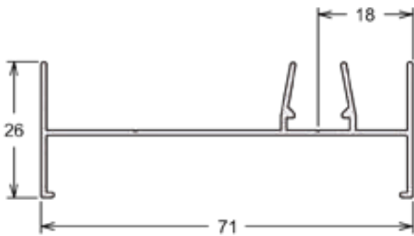
SU-003 | PESO: 2,700 KG/BR Marco Lateral Vertical
