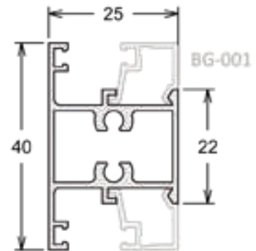
25-026 | PESO: 2,900 KG/BR Travessa Horizontal - 40mm
