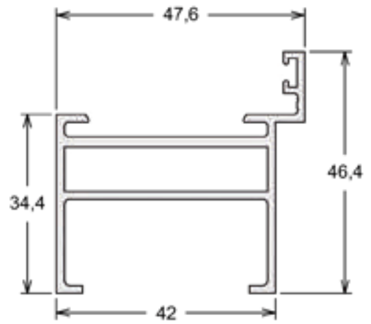
P-280 | PESO: 5,000 KG/BR Marco Tubular - Porta de Giro
