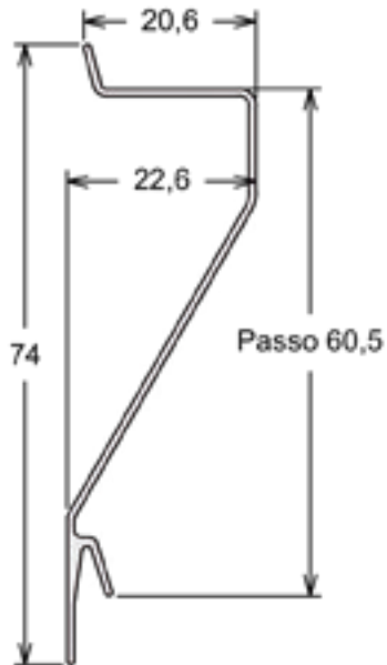
VZ-006 | PESO: 1,650 KG/BR Veneziana
