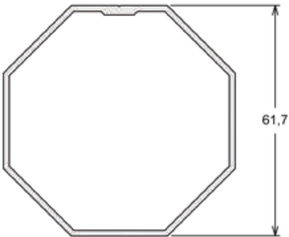
IT-008 | PESO: 5,400 KG/BR Tubo Recolhedor - 60mm
