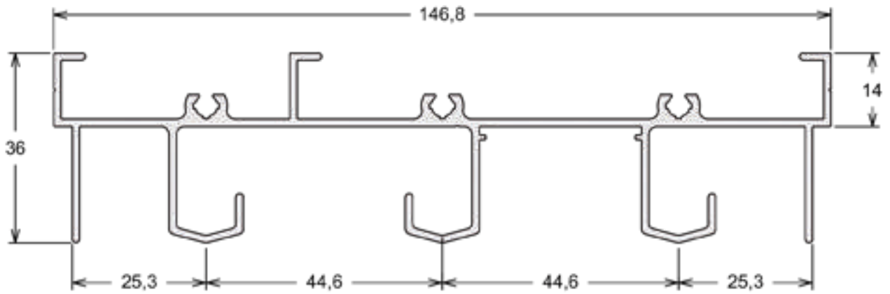
LG-062 | PESO: 9,600 KG/BR Marco Superior Horizontal
