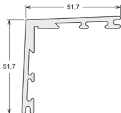
CL-006 | PESO: 3,200 KG/BR - 3 METROS Cantoneira de Ligação 45°
