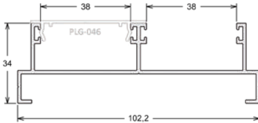
LG-045 | PESO: 5,400 KG/BR Marco Lateral Vertical
