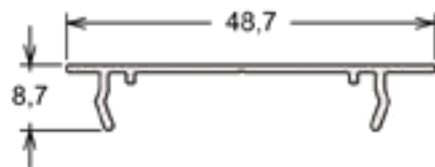
LG-046 | PESO: 1,300 KG/BR Tampa do Marco Lateral
