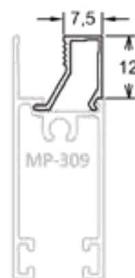
BG-202 | PESO: 0,600 KG/BR
