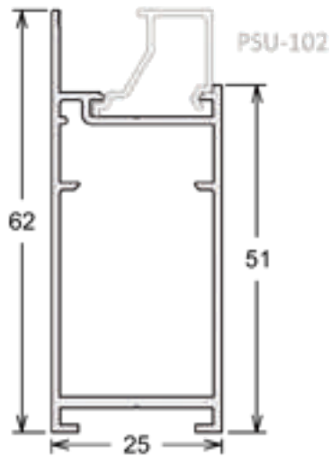
SU-211 | PESO: 3,400 KG/BR Folha Lateral e Superior - Porta de Giro
