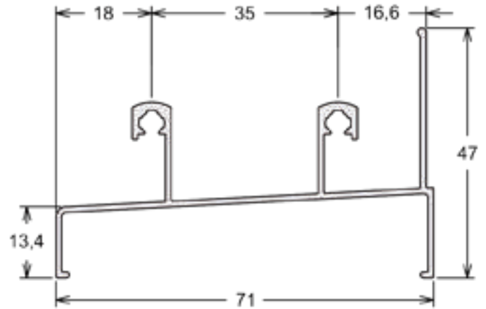
SU-002 | PESO: 3,700 KG/BR Marco Superior Horizontal
