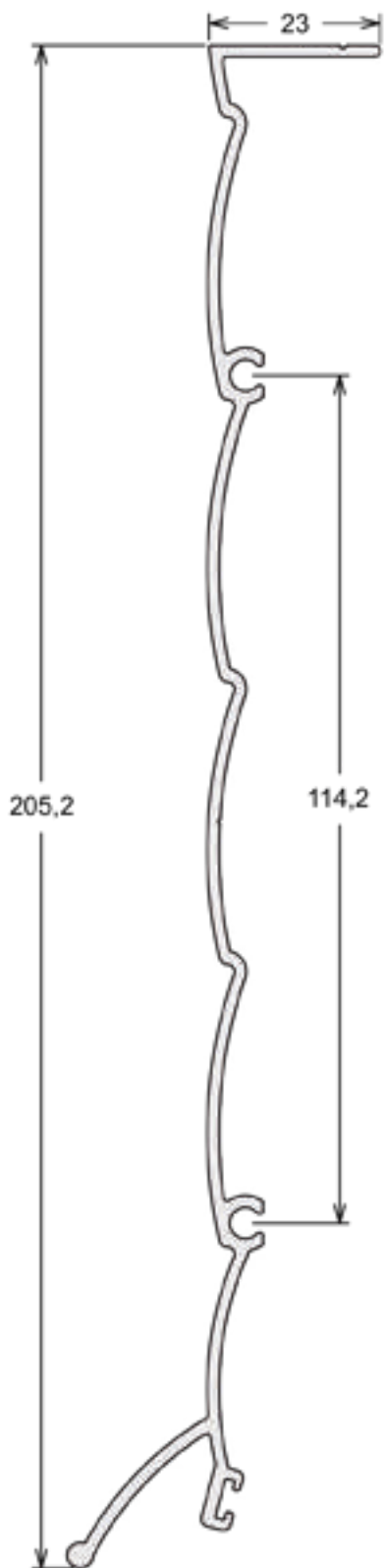
MN-039 | PESO: 7,100 KG/BR Tampa Externa Horizontal
