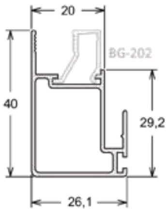
MP-302 | PESO: 2,500 KG/BR Folha Mão de Amigo Externo
