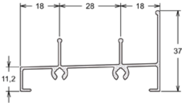
MP-358 | PESO: 3,300 KG/BR Marco Inferior Horizontal
