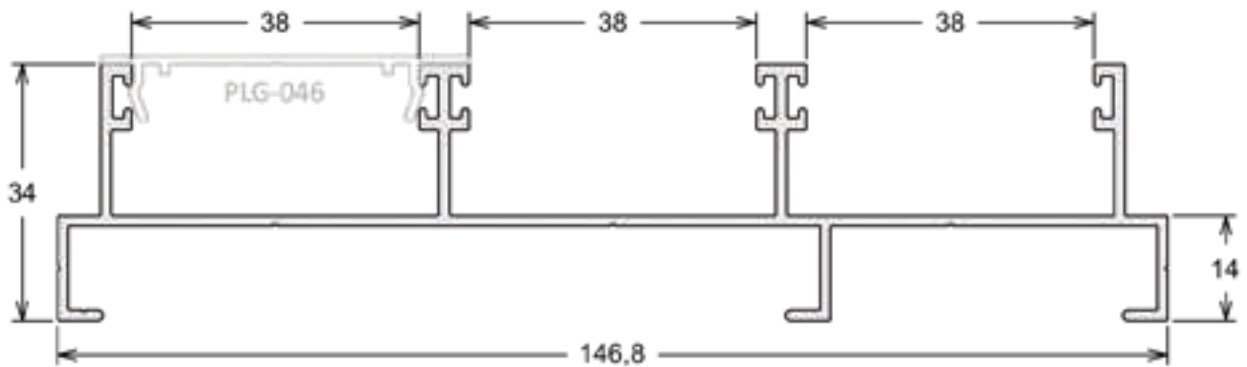
LG-064 | PESO: 7,500 KG/BR Marco Lateral Vertical
