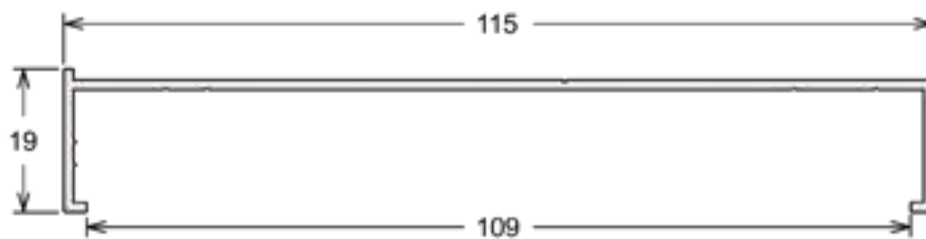
IT-010 | PESO: 3,300 KG/BR
