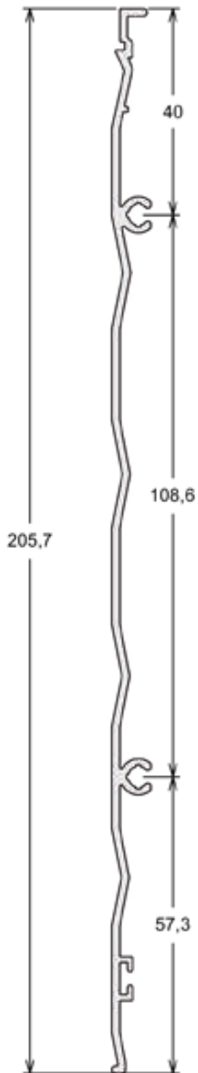
IT-015 | PESO: 6,100 KG/BR Tampa Externa Horizontal
