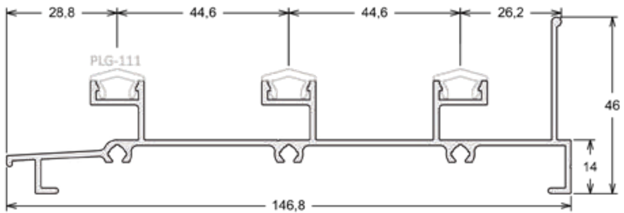
LG-116 | PESO: 8,300 KG/BR Marco Inferior Horizontal
