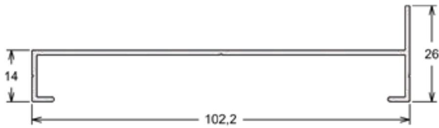
LG-002 | PESO: 3,300 KG/BR Marco Lateral Vertical
