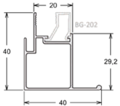
MP-321 | PESO: 2,500 KG/BR Folha Mão de Amigo Interno - Com Reforço
