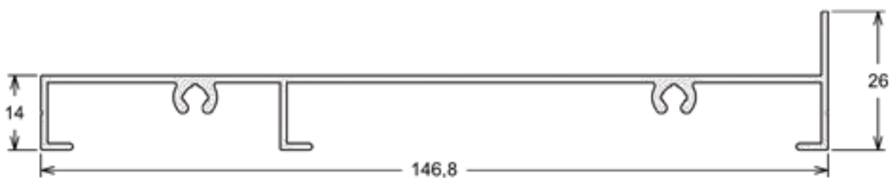
LG-116 | PESO: 8,300 KG/BR Marco Inferior Horizontal
