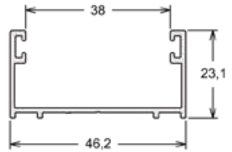
LG-028 | PESO: 2,300 KG/BR Complemento do Marco Lateral
