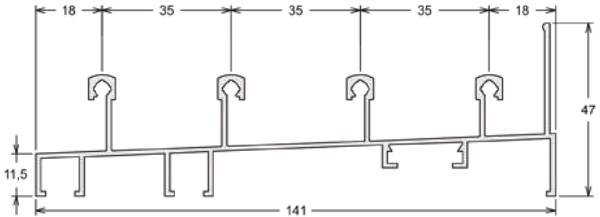
SU-122 | PESO: 8,300 KG/BR Marco Inferior Horizontal 4 Folhas
