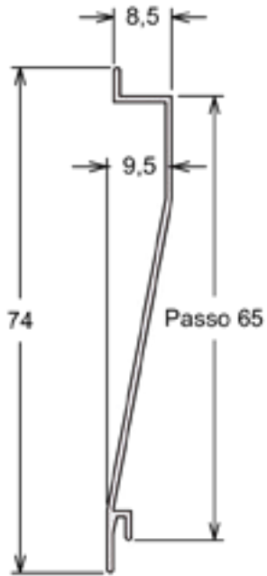
VZ-024 | PESO: 1,400 KG/BR Veneziana
