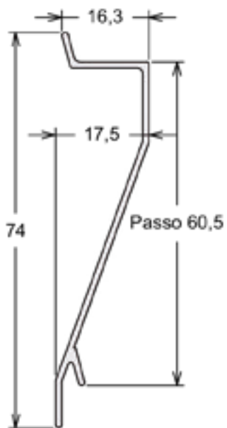
VZ-023 | PESO: 2,000 KG/BR Veneziana
