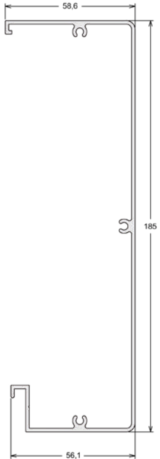
LG-230 | PESO: 9,500 KG/BR Tampa Interna Horizontal
