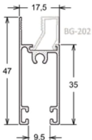
MP-309 | PESO: 2,300 KG/BR
