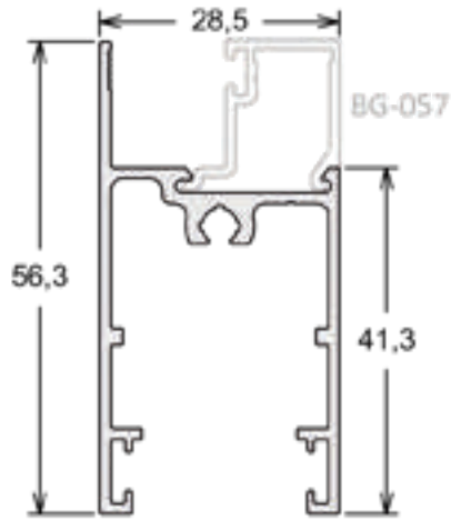
LG-006 | PESO: 3,600 KG/BR
