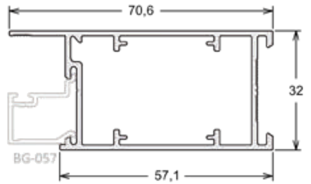
LG-043 | PESO: 5,300 KG/BR
