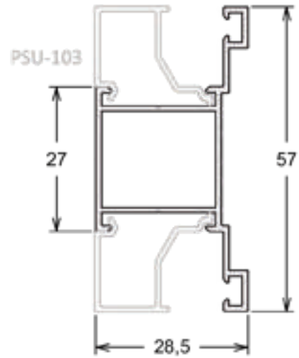
SU-085 | PESO: 2,700 KG/BR Tubo Recolhedor - 60mm
