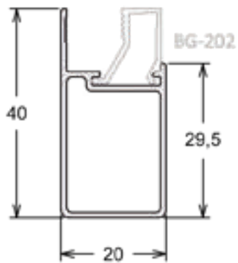
MP-300 | PESO: 1,900 KG/BR Folha Lateral Vertical
