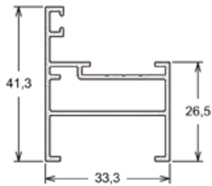
SU-279 | PESO: 3,100 KG/BR Marco Tubolar - Porta de Giro
