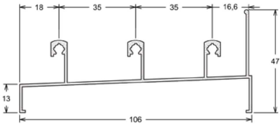
SU-011 | PESO: 5,500 KG/BR
