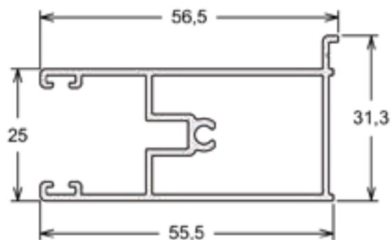
MN-007 | PESO: 4,000 KG/BR Guia da Persiana
