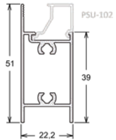
SU-211 | PESO: 3,400 KG/BR Folha Lateral e Superior - Porta de Giro
