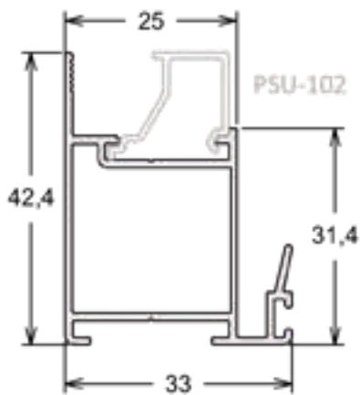
SU-041 | PESO: 2,800 KG/BR Folha Mão de Amigo Externo
