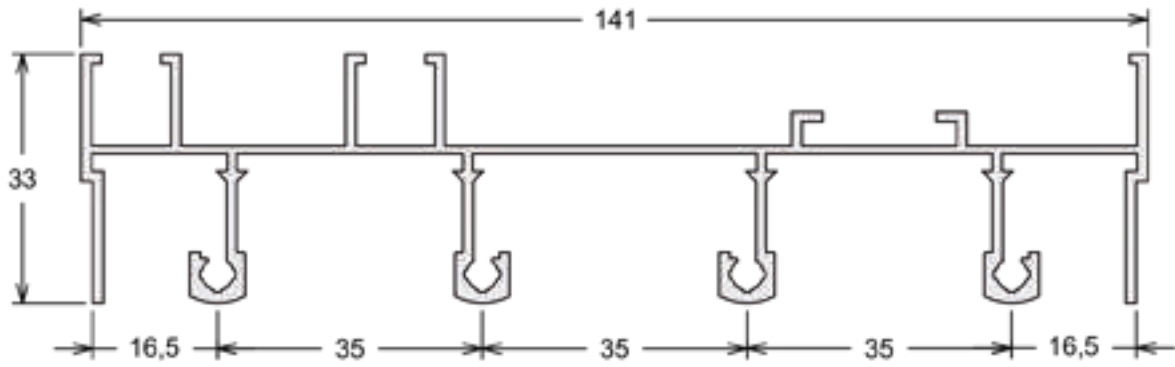
SU-121 | PESO: 8,600 KG/BR Marco Superior Horizontal 4 Folhas
