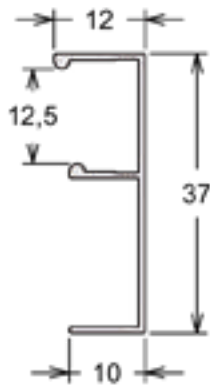
MP-347 | PESO: 1,000 KG/BR Arremate / Vista Interna
