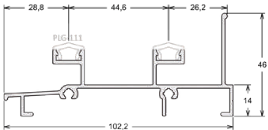
LG-159 | PESO: 6,000 KG/BR Marco Inferior Horizontal
