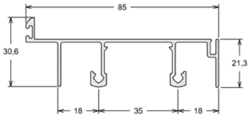
IT-002 | PESO: 4,700 KG/BR Travessa Intermediária - Integrada
