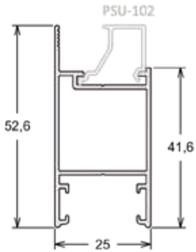
SU-039 | PESO: 3,000 KG/BR Folha Lateral Vertical
