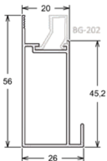
MP-070 | PESO: 3,100 KG/BR
