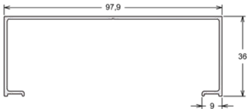
MN-050 | PESO: 4,000 KG/BR Marco Lateral Vertical
