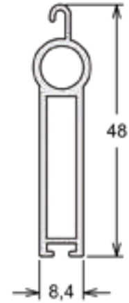
IT-009 | PESO: 2,500 KG/BR Terminal da Persiana
