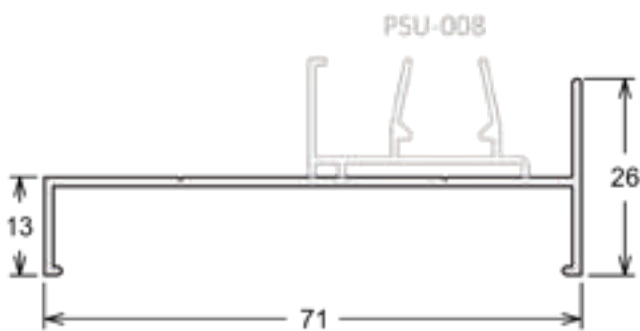
SU-007 | PESO: 2,200 KG/BR Marco Vertical
