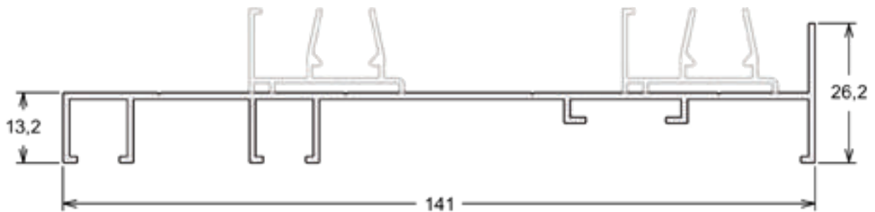
SU-123 | PESO: 4,900 KG/BR Marco Lateral Vertical
