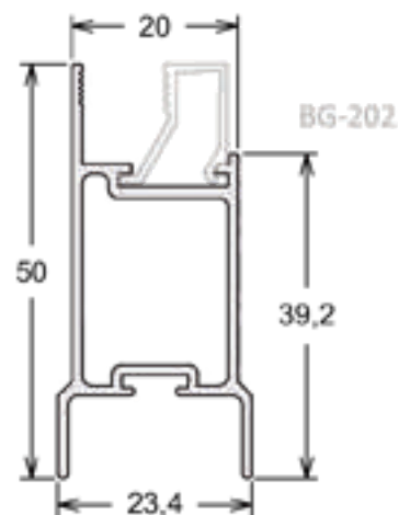
MP-318 | PESO: 2,800 KG/BR Folha Lateral Vertical
