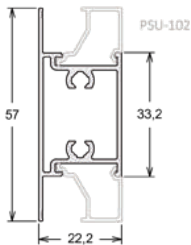
SU-227 | PESO: 3,300 KG/BR
